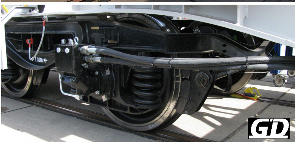
Drehgestell mit Zusatzeinrichtung: Railcare rCe Powerpack, gesehen unter 33 RIV 80 D-AAEC 4925 602-3 Sggmrs 90'.S23 Freight Car Bogie with additional device: Railcare rCe Powerpack, seen with 33 RIV 80 D-AAEC 4925 602-3 Sggmrs 90'.S23
