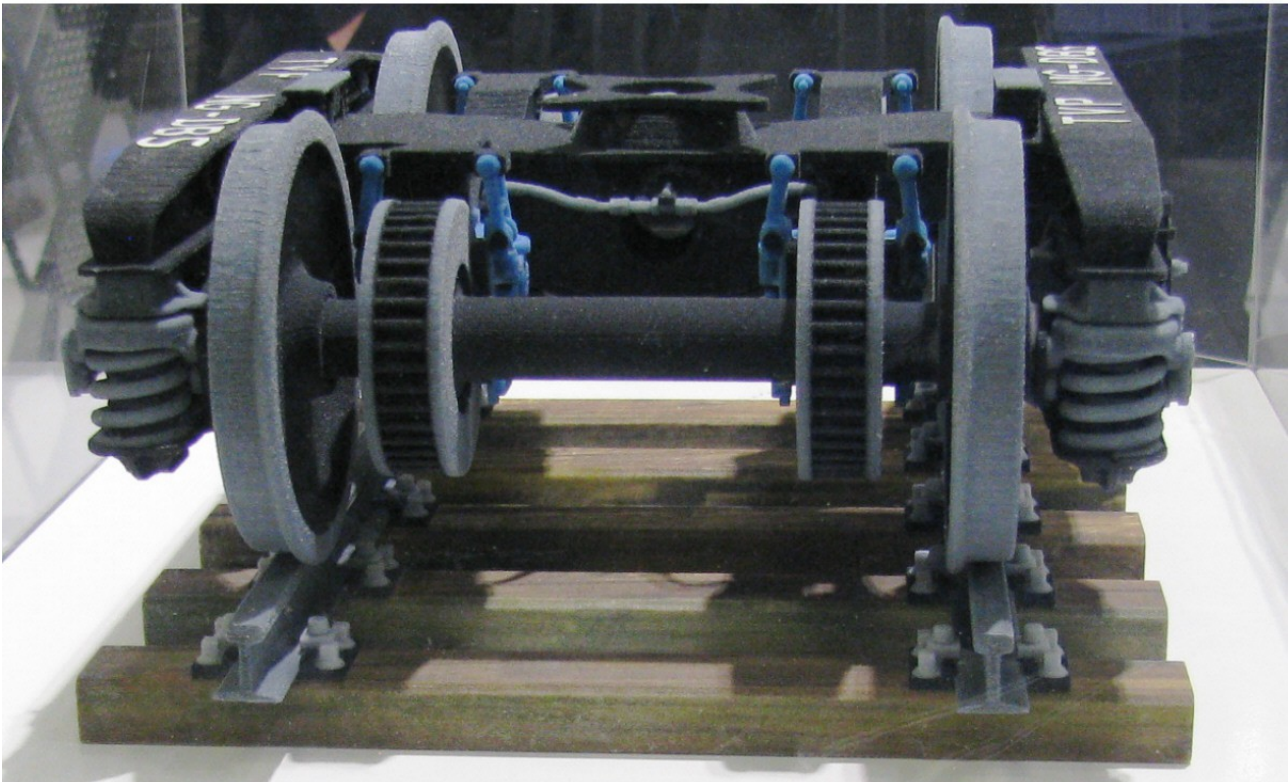
Güterwagen-Drehgestell/Freight Car Bogie TVP NG-DBS (ohne Kopfstücke, mit Radsatzkopplung und Scheibenbremsen/without head beams, but with wheelset coupling and disk brakes)
